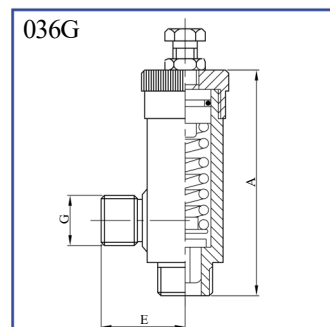
Pojistný ventil s vnějšími závit AISI 316L
