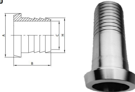
Hadicový nástavec dle DIN s kuželovým hrdlem dle DIN 11851 AISI 304/L, AISI 316/L
