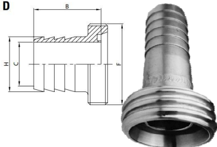
Hadicový nástavec dle DIN se závitovým hrdlem dle DIN 11851 AISI 304/L, AISI 316/L
