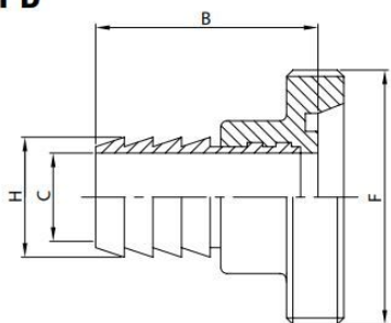
Hadicový nástavec dle SMS se závitovým hrdlem dle DIN 11851 AISI 304/L, AISI 316/L
