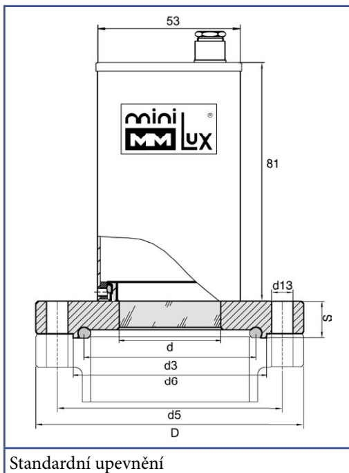
Osvětlení série miniLUX STERI-LINE, typ BKVLR LED DA, 24V, připevněno k průhledítku dle DIN 11864-2, DN 50
