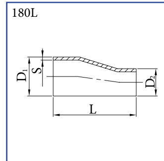
Redukce excentrická DIN-1 přivařovací - dlouhá AISI 304/L, AISI 316/L
