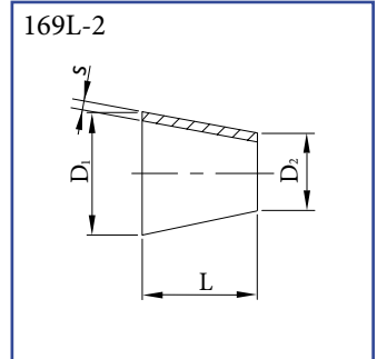
Redukce souosá DIN řada 2 přivařovací - krátká AISI 304/L, AISI 316/L
