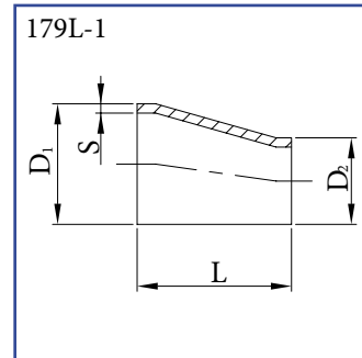
Redukce excentrická DIN-1 přivařovací - krátká AISI 304/L, AISI 316/L
