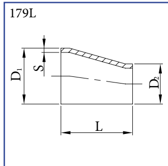
Redukce excentrická DIN-1 přivařovací AISI 304/L, AISI 316/L
