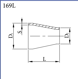
Redukce souosá DIN řada 1 přivařovací AISI 304/L, AISI 316/L
