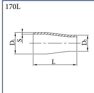
Redukce souosá DIN řada 1 přivařovací - dlouhá AISI 304/L, AISI 316/L
