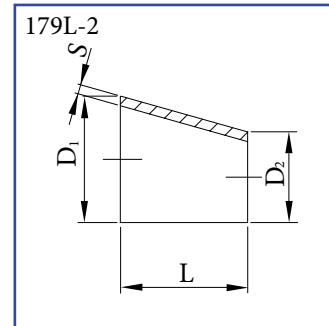
Redukce excentrická DIN-2 přivařovací - krátká AISI 304/L, AISI 316/L
