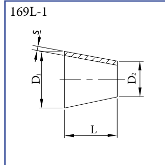
Redukce souosá DIN řada 1 přivařovací - krátká AISI 304/L, AISI 316/L
