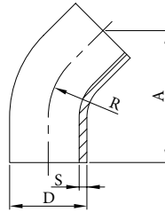
Koleno 45° dlouhé SMS pro orbitální svařování AISI 304/L, AISI 316/L
