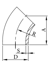
Koleno 45° krátké DIN řada 2 přivařovací AISI 304/L, AISI 316/L
