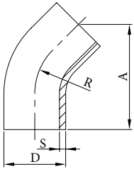
Koleno 45° dlouhé DIN řada 1 pro orbitální svařování AISI 304/L, AISI 316/L
