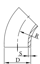
Koleno 45° krátké ISO přivařovací AISI 304/L, AISI 316/L
