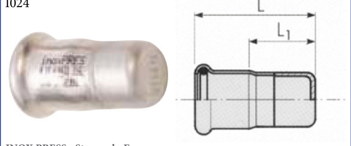
INOX PRESS - Stop end - F
