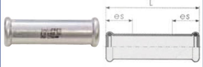
INOX PRESS - Slip coupling - F/F
