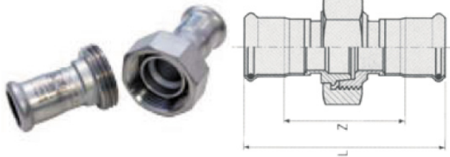
INOX PRESS - Conical union - F/F
