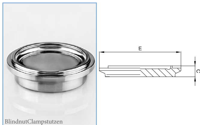
Aseptic Clamp with groove DIN 11864-1-A and DIN 11853-1
