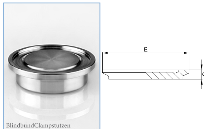
Aseptic Clamp with collar DIN 11864-1-A a DIN 11853-1
