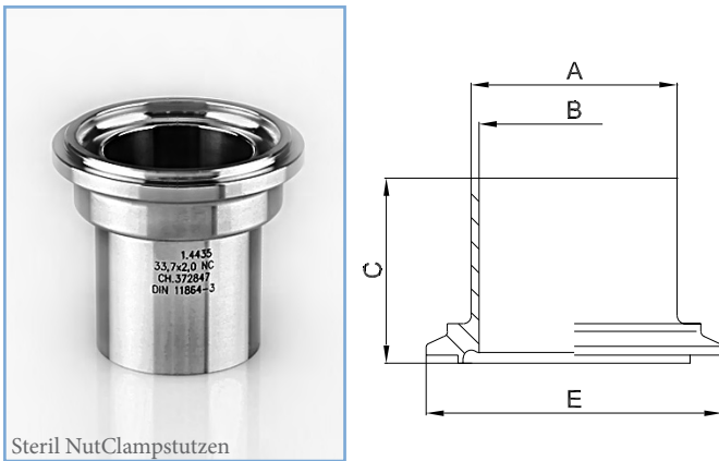
Aseptic Clamp with groove DIN 11864-3-A:
