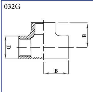
T-kus F/F/F s vnitřními závit AISI 316 (AISI 304)
