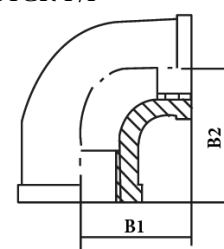
Koleno 90° redukované s vnitřními závity AISI 316
