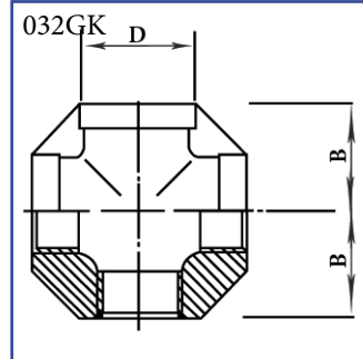
Kříž F/F/F/F s vnitřními závit AISI 316
