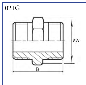
Dvounipl se šestihrannem AISI 316
