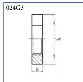
Šestihranná matka s vnitřním závitem AISI 316 (AISI 304)
