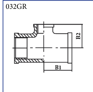
T-kus redukovaný F/F/F s vnitřními závit AISI 316
