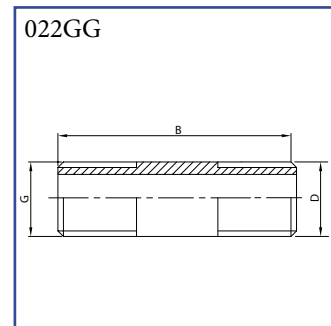
Trubkový dvounipl AISI 316
