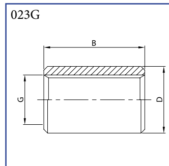
Nátrubek s vnitřním závitem (Mufna) AISI 316
