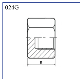
Šestihranná zátka s vnitřním závitem AISI 316
