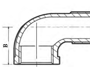
Koleno 90° vnitřní / vnější závit AISI 316 (AISI 304)
