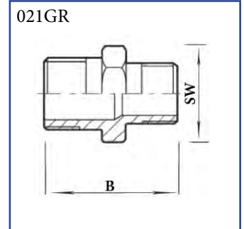
Redukovaný dvojnopl se šestihrannem AISI 316 (AISI 304)
