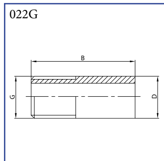
Nátrubek s vnějším závitem přivařovací (Nipl) AISI 316
