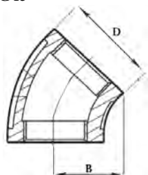
Koleno 45° s vnitřními závity AISI 316
