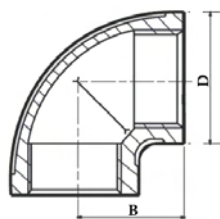
Koleno 90° s vnitřními závity AISI 316 (AISI 304)
