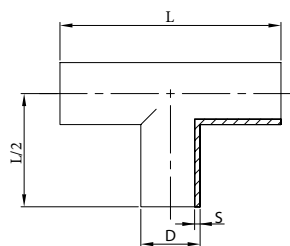
T-kus dlouhý SMS přivařovací AISI 304/L, AISI 316/L
