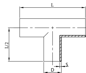
T-kus dlouhý ISO přivařovací AISI 304/L, AISI 316/L
