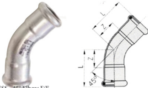
INOX PRESS - 45° Elbow F/F
