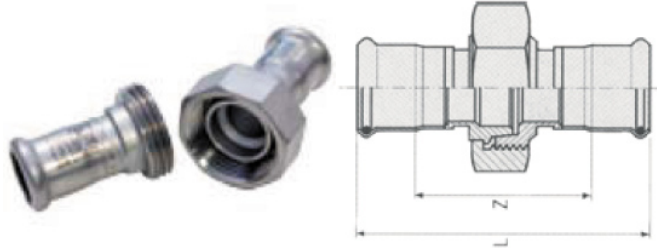
INOX PRESS - Conical union - F/F
