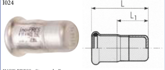
INOX PRESS - Stop end - F
