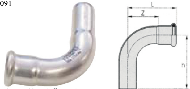
INOX PRESS - 90° Elbow M/F
