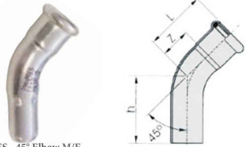
INOX PRESS - 45° Elbow M/F
