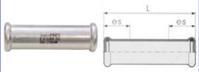
INOX PRESS - Slip coupling - F/F
