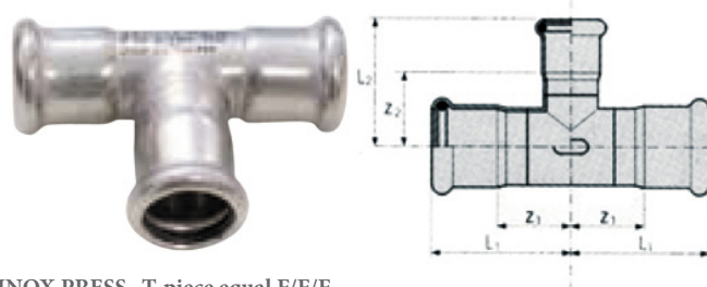
INOX PRESS T-piece equal F/F/F
