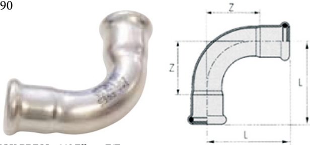
INOX PRESS - 90° Elbow F/F
