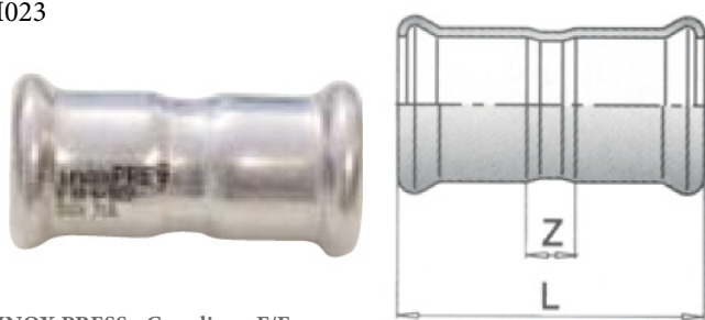
INOX PRESS - Coupling - F/F
