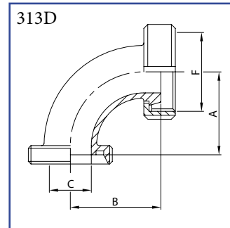
Koleno 90° DIN závit / kužel. hrdlo s maticí AISI 304/L, AISI 316/L
