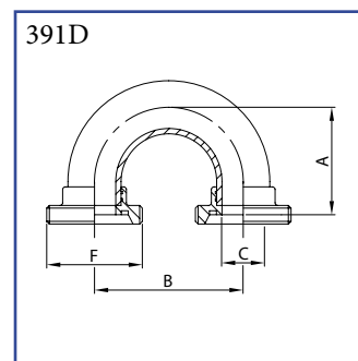
Koleno 180° DIN se závitovými konci AISI 304/L, AISI 316/L
