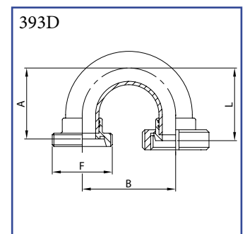
Koleno 180° DIN závit / kužel. hrdlo s maticí AISI 304/L, AISI 316/L
