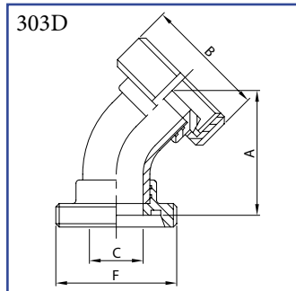
Koleno 45° DIN závit / kužel. hrdlo s maticí AISI 304/L, AISI 316/L
