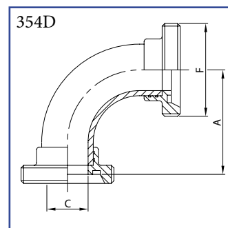
Koleno 90° dlouhé DIN se závitovými konci AISI 304/L, AISI 316/L
