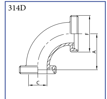
Koleno 90° DIN se závitovými konci AISI 304/L, AISI 316/L
