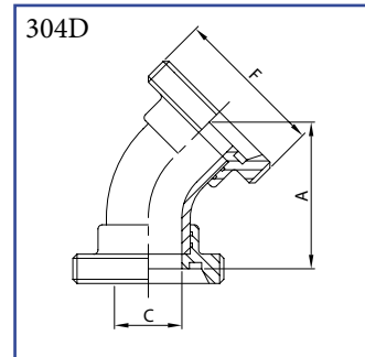
Koleno 45° DIN se závitovými konci AISI 304/L, AISI 316/L
