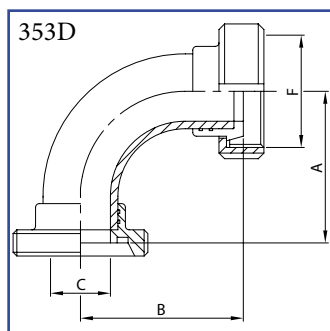
Koleno 90° dlouhé DIN závit / kužel. hrdlo s maticí AISI 304/L, AISI 316/L
