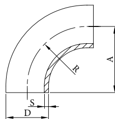
Koleno 90° SMS přivařovací AISI 304/L, AISI 316/L
