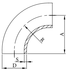
Koleno 90° DIN řada 1 přivařovací AISI 304/L, AISI 316/L
