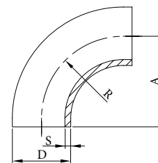
Koleno 90° ISO přivařovací AISI 304/L, AISI 316/L
