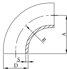
Koleno 90° DIN řada 2 přivařovací AISI 304/L, AISI 316/L
